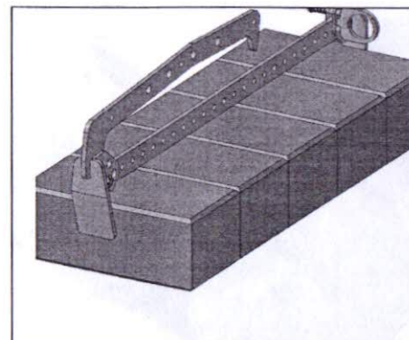
Рисунок 2.1 – Общий вид захвата поперечно расположенной плитки общим габаритом 240x120xh
