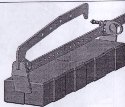
Рисунок 3.2 – Общий вид захвата продольно расположенной плитки общим габаритом 250x125xh.
