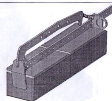
Рисунок 2.2 – Общий вид захвата продольно расположенной плитки общим габаритом 240x120xh.
