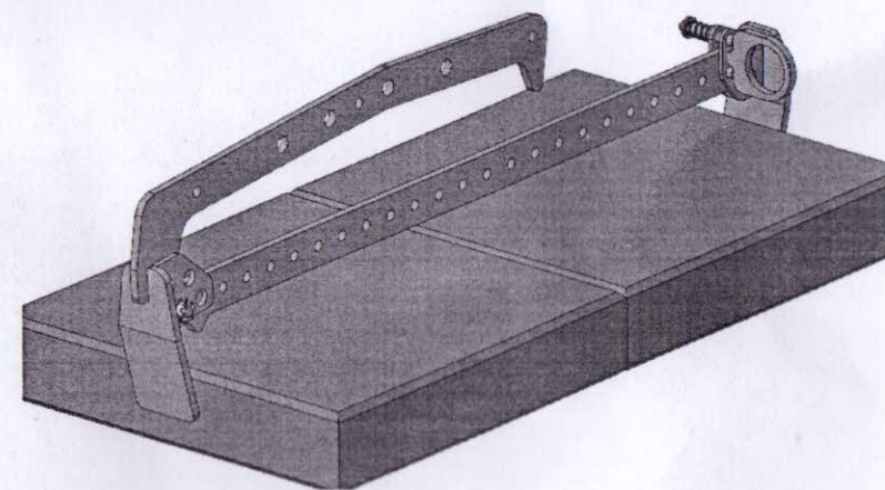
Рисунок 4.1 – Общий вид захвата плитки общим габаритом 300x300xh.
