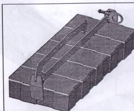
Рисунок 3.1 – Общий вид захвата поперечно расположенной плитки общим габаритом 250x125xh
