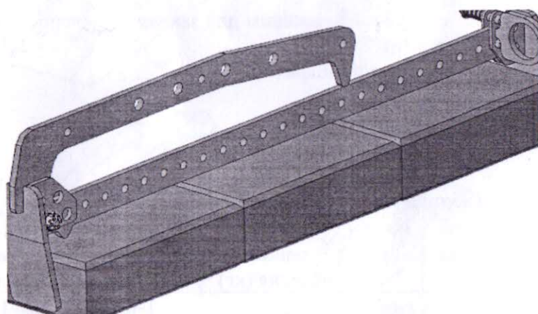
Рисунок 1.2 – Общий вид захвата продольно расположенной плитки общим габаритом 200x100xh.
