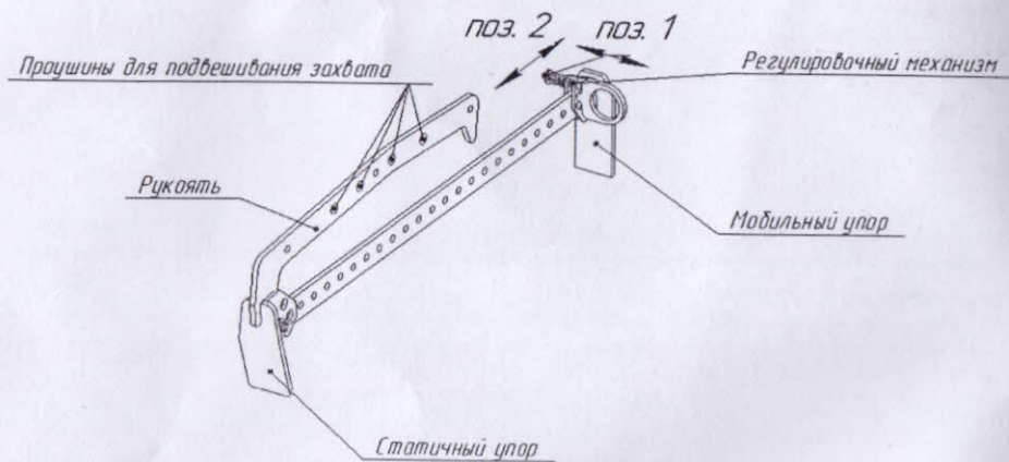
Рисунок – 1. Общий вид захвата ручного плиточного.
