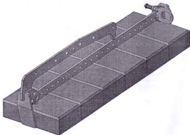
Рисунок 1.1 – Общий вид захвата поперечно расположенной плитки общим габаритом 200x100xh.
