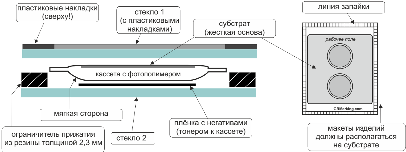
Рис.9а Фотополимерная кассета: расположение в рамке
