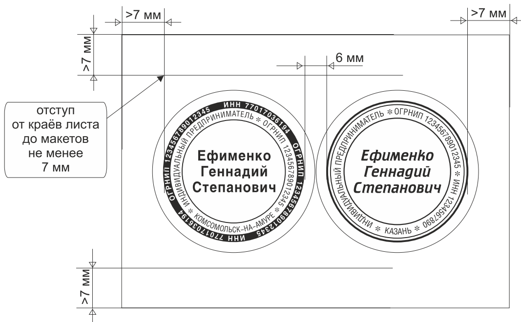
Рис.2b Расположение нескольких макетов на листе
