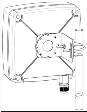
Монтаж антенны
