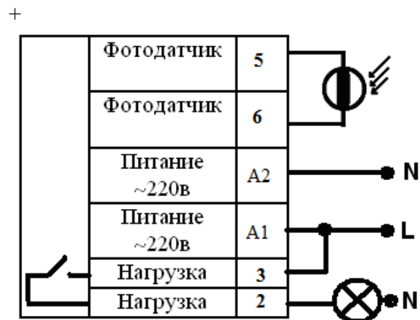
Рис.3. Типовая схема подключения фотореле к сети 220в.
