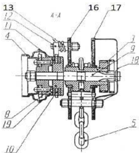
Рис. 2 Разрез механизма тали
