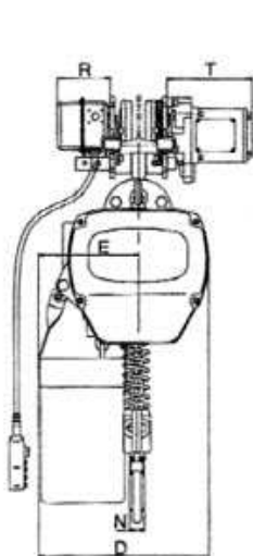
Рисунок 1. Габаритные размеры ННВД-Т 0,5 – 5т.
