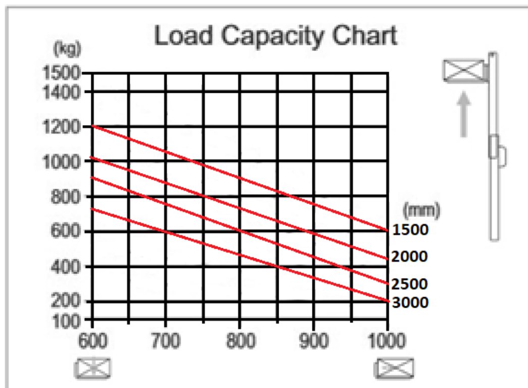
График грузоподъемности
