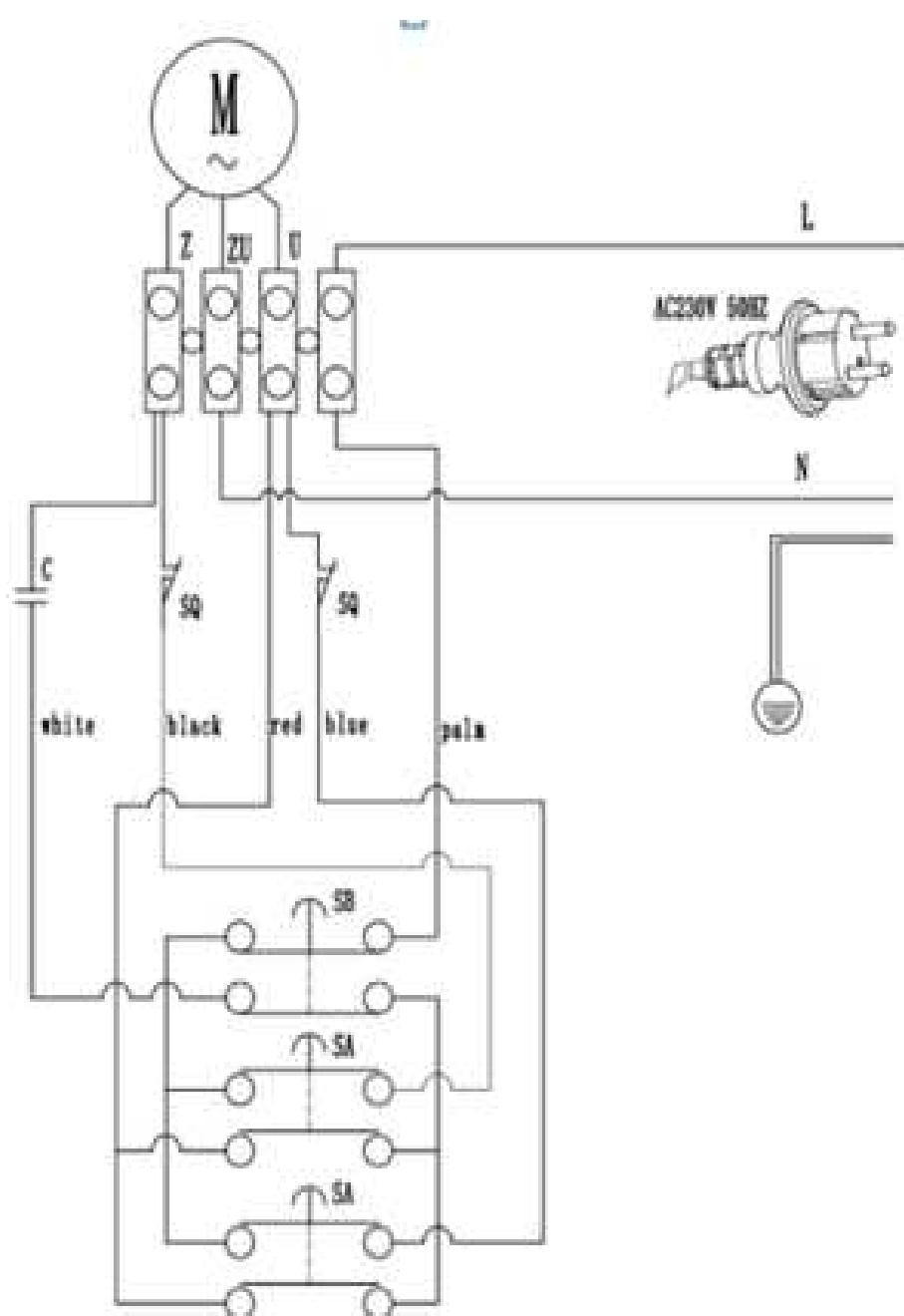
Схема электрическая
