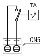
регулятор комнатной температуры
