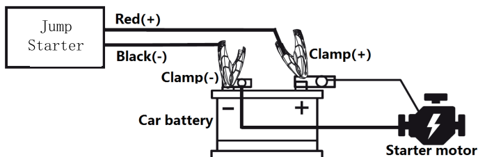
Рис. 2: Восстановление соединения клемм с аккумулятором автомобиля.
