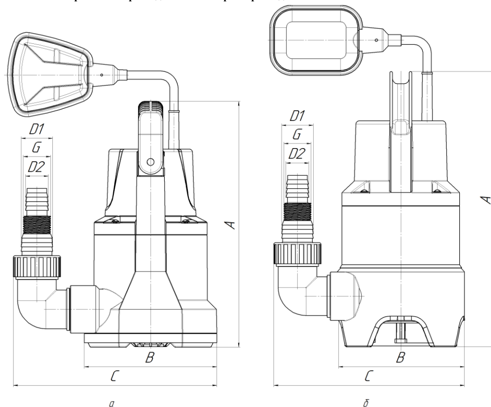
Рисунок 6 – Габаритные и присоединительные размеры изделия
