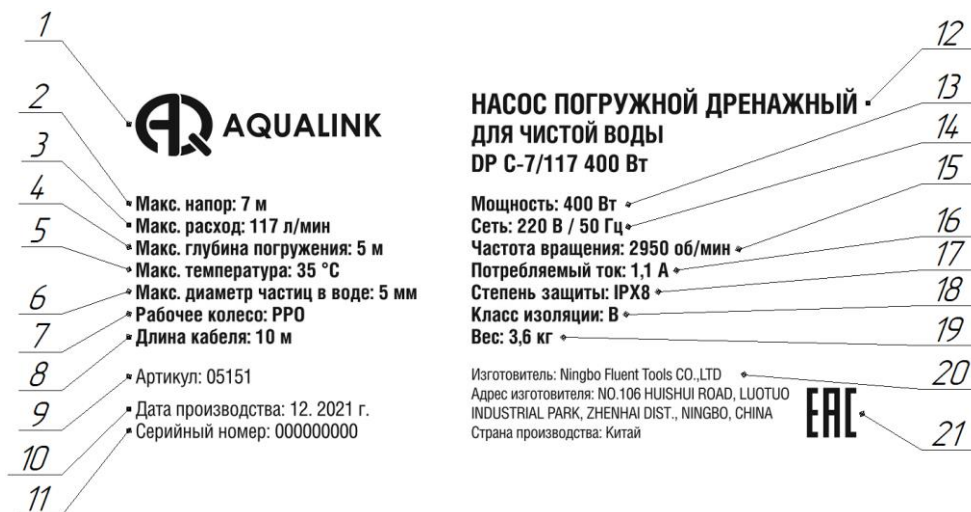
Рисунок 1 – Шильдик изделия
