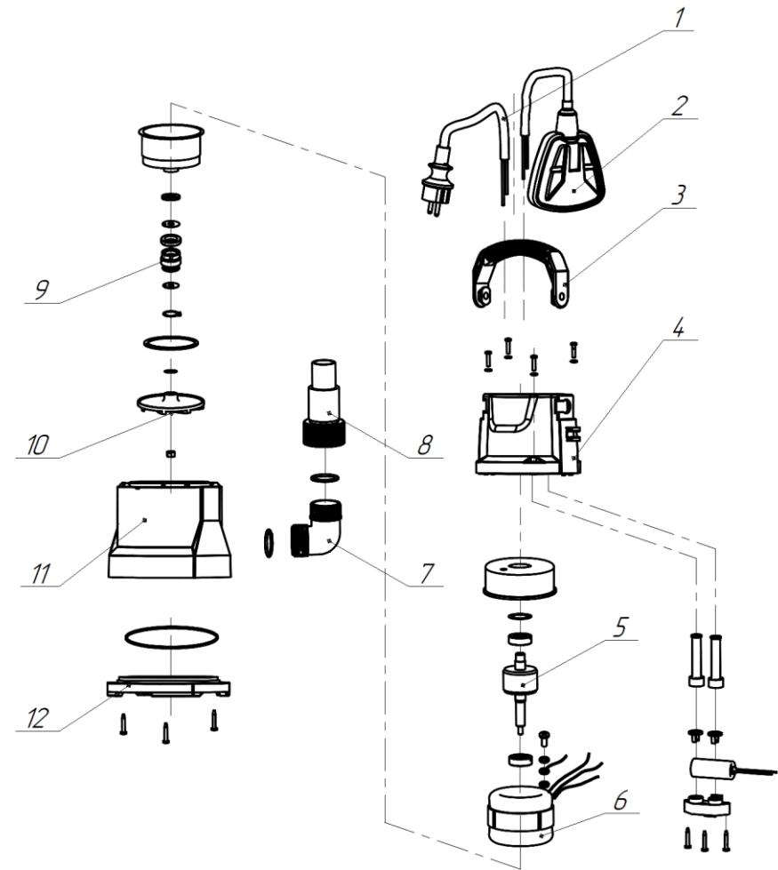
Рисунок 4 – Общий вид и конструкция насоса для чистой воды
