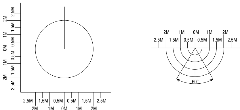
– Рисунок 5 – Диаграммы направленности для встроенного датчика движения
