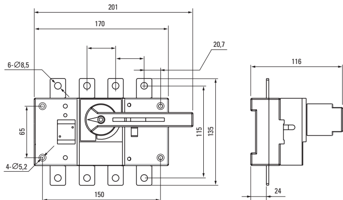
Рисунок 1б - Монтажные размеры рубильника PowerSwitch 160 А четырехполюсного
