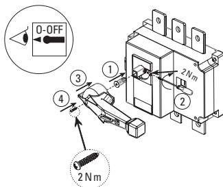
Рисунок 7а - Монтаж ручки на корпус рубильников 160-630 А
