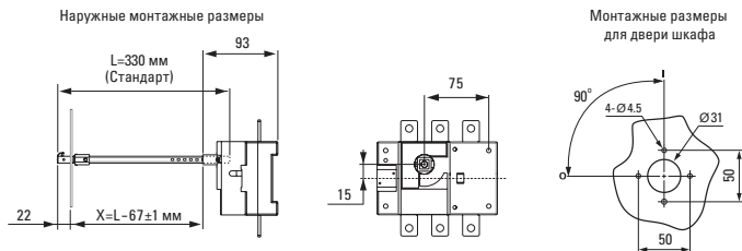
Рисунок 9б - Монтажные размеры при установке на дверцу шкафа для рубильников 160 А
