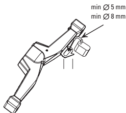
Рисунок 8б - Блокировка ручки рубильников 1000-1600 А навесным замком
