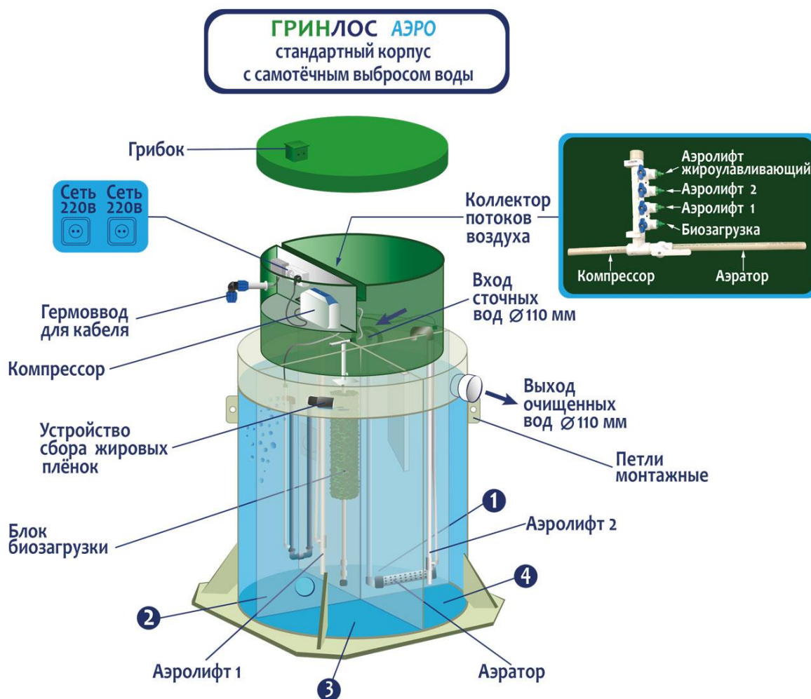
Рисунок 1. Схема модели с самотечным сбросом сточных вод и стандартным корпусом
