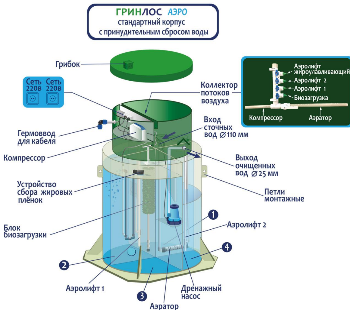
Рисунок 3. Схема модели с принудительным сбросом сточных вод и стандартным корпусом
