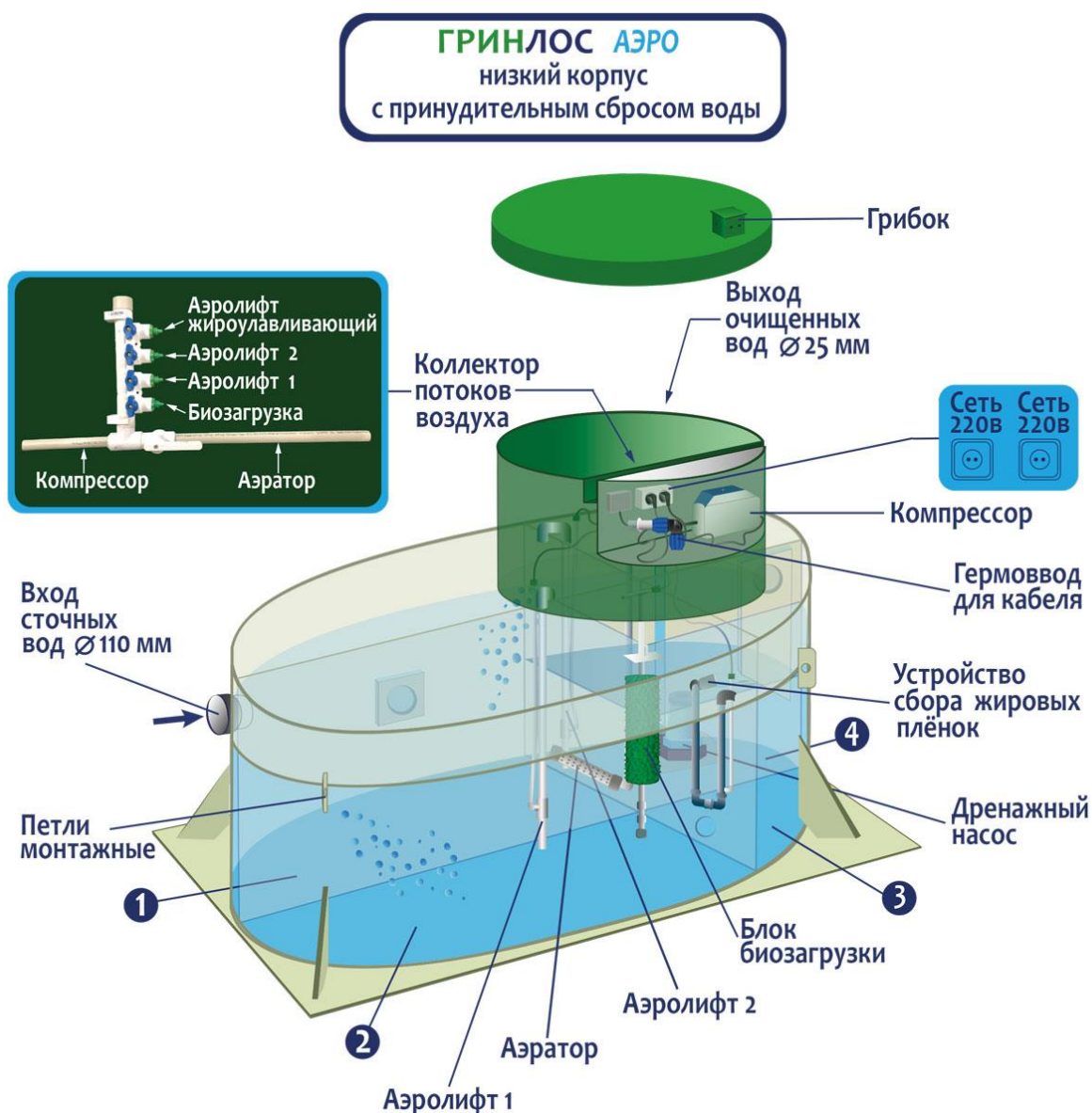
Рисунок 4. Схема модели с принудительным сбросом сточных вод и низким корпусом
