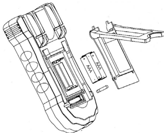
Рисунок 4. Замена батареи и предохранителей
