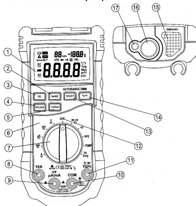
Рисунок 1. Схема мультиметра
