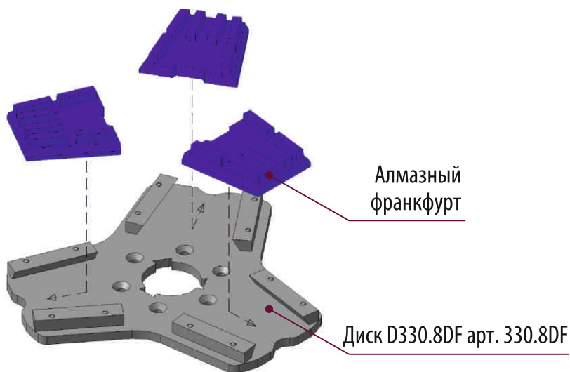
Рис. 15 Установка алмазных франкфуртов
