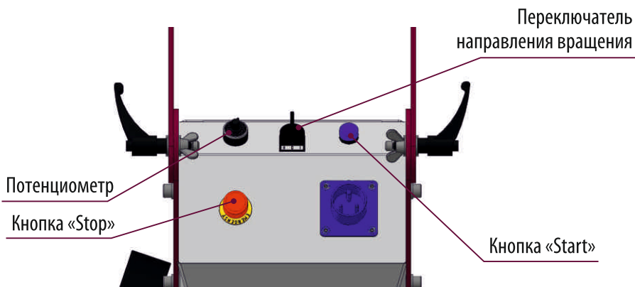
Рис. 4 Схема расположения кнопок управления
