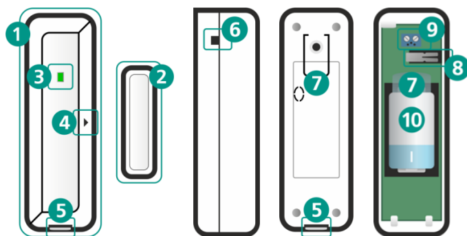
Рисунок 2.1 – Внешний вид датчика
