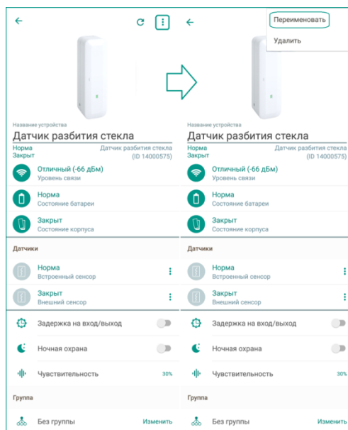
Рисунок 12.3 – Вызов меню на экране настройки датчика
