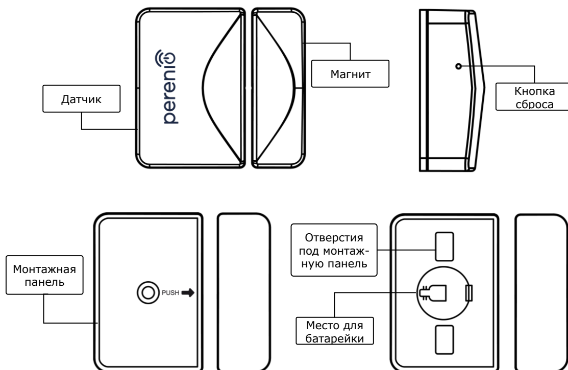
Рисунок 11 – Составные части датчика открытия PECWS01
