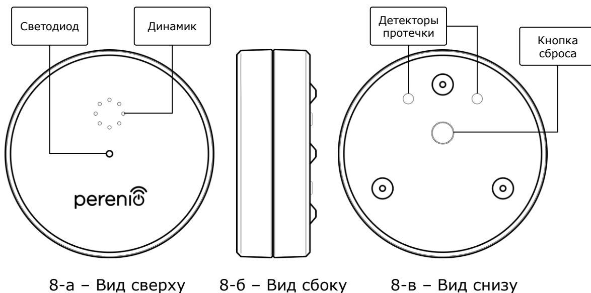
Рисунок 8 – Кнопки и компоненты датчика протечки PECLS01
