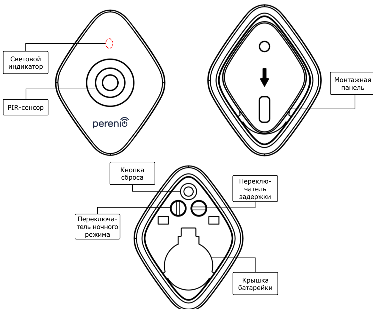
Рисунок 14 – Составные части датчика движения PECMS01
