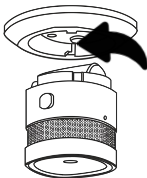
Рисунок 6 – Отсоединение монтажного кронштейна от корпуса датчика дыма
