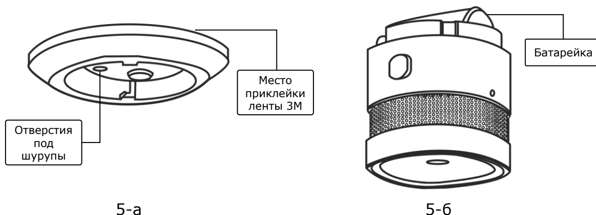
Рисунок 5 – Крепление датчика дыма на шурупы или ленту 3М
