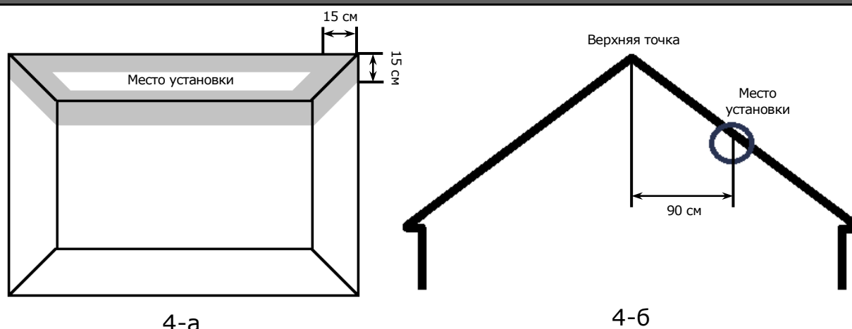
Рисунок 4 — Установка датчика дыма на плоский/скошенный потолок
