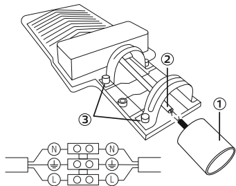
Рис. 1. Монтаж светильника
