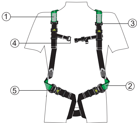
Вид спереди
