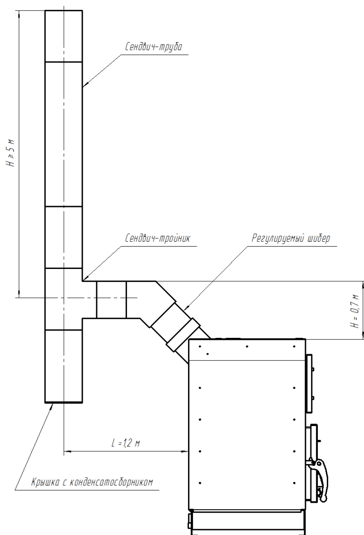
Рисунок 5.2 – Подключение котла к дымовой трубе
