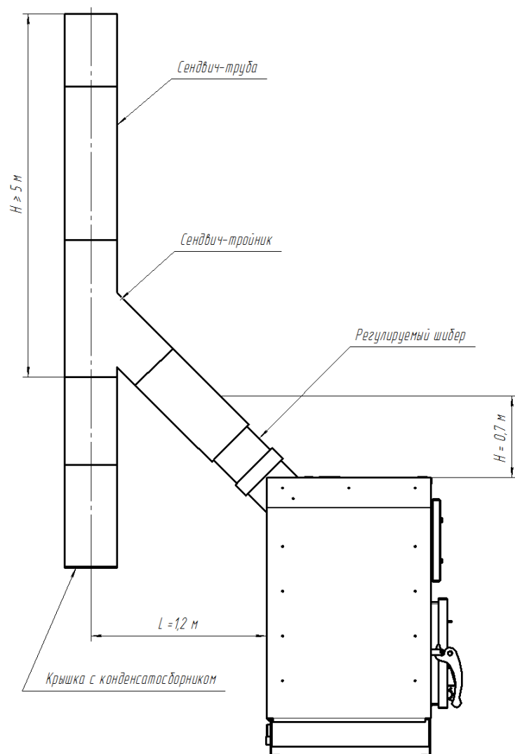
Рисунок 5.3 – Подключение котла к дымовой трубе
