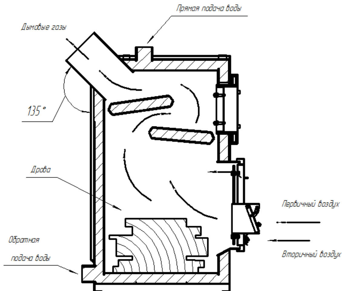
Рисунок 1 – Схема КОД-12
