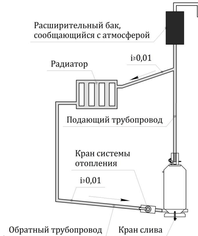
Рисунок 7 – Схема открытой системы отопления с естественной циркуляцией
