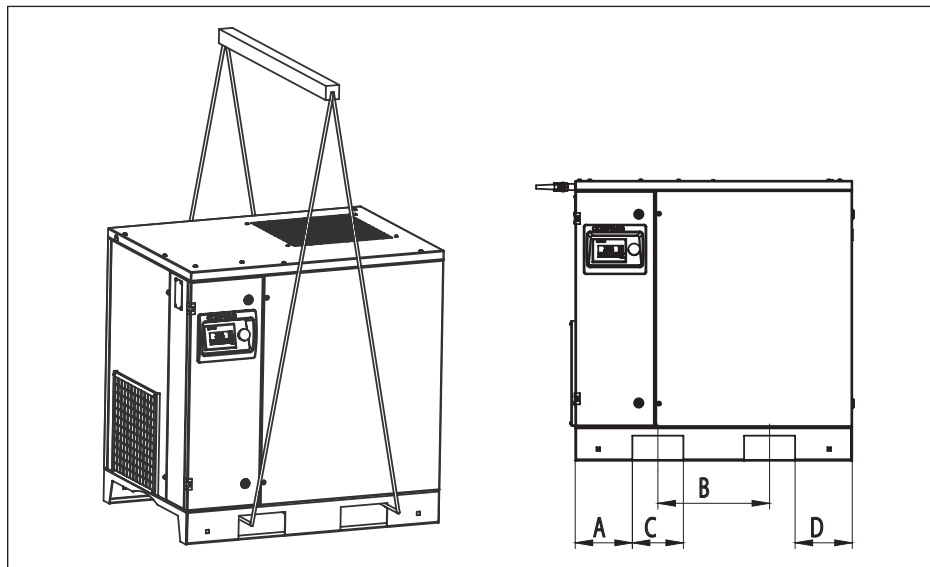
Рис. 3.1.1.1. Схема для такелажных работ F05.. – F22.
