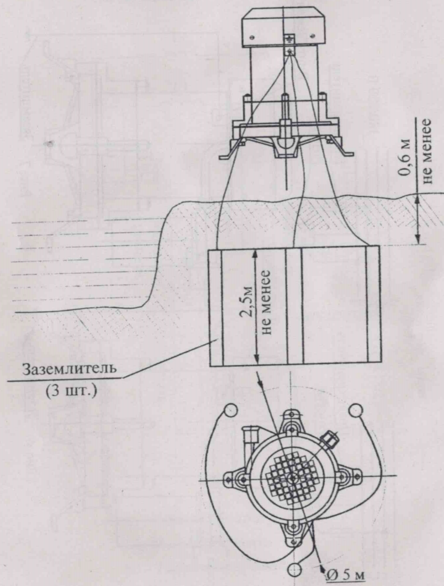
Схема заземления
