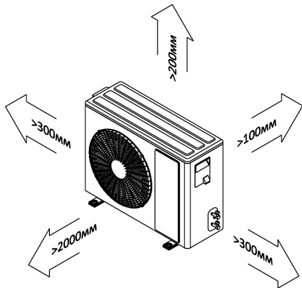
Установочные размеры наружн блок
