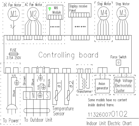
Внутренний блок моделей RAS/RAC-V09N2X, V12N2X, V18N2X, V24N2X
