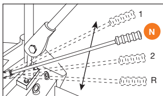
Коробка передач
