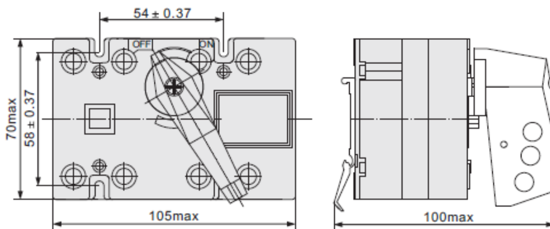
Габаритные и установочные размеры BP-101 (W) 40-63A, 3P(4P)
