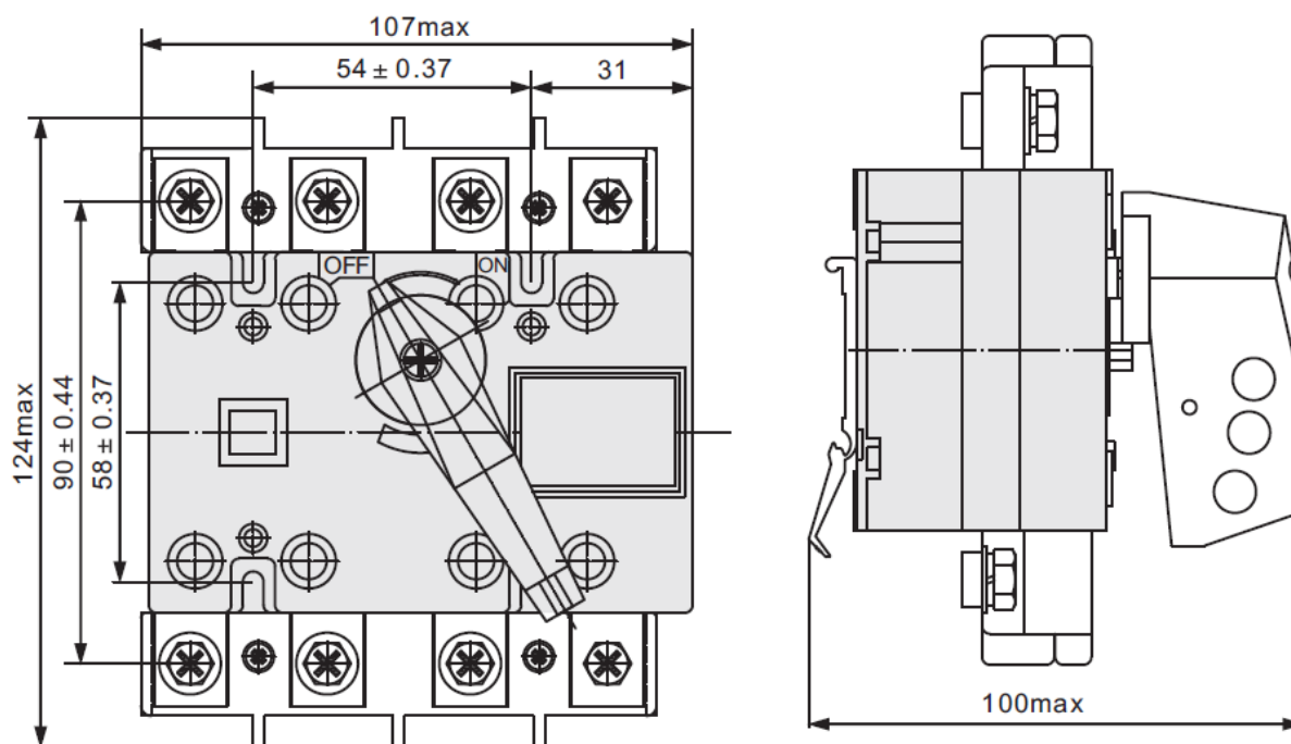
Габаритные и установочные размеры BP-101 (W) 80-100, 3P(4P)
