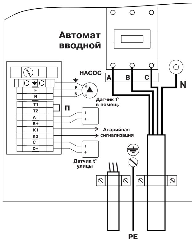
Рис.3 Схема подключения электроводонагревателя
