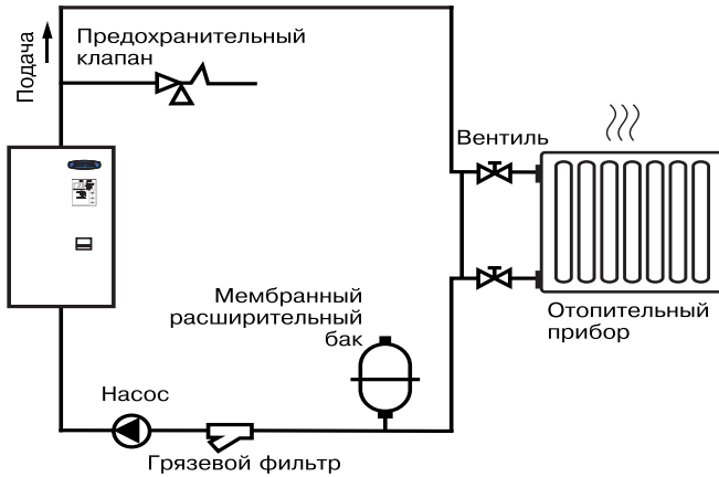
Рис.10 Упрощенная схема подключения электроводонагревателя в отопительную систему с циркуляционным насосом
