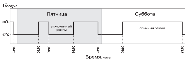
Рис.8 График температуры воздуха в помещении для Режим 3
