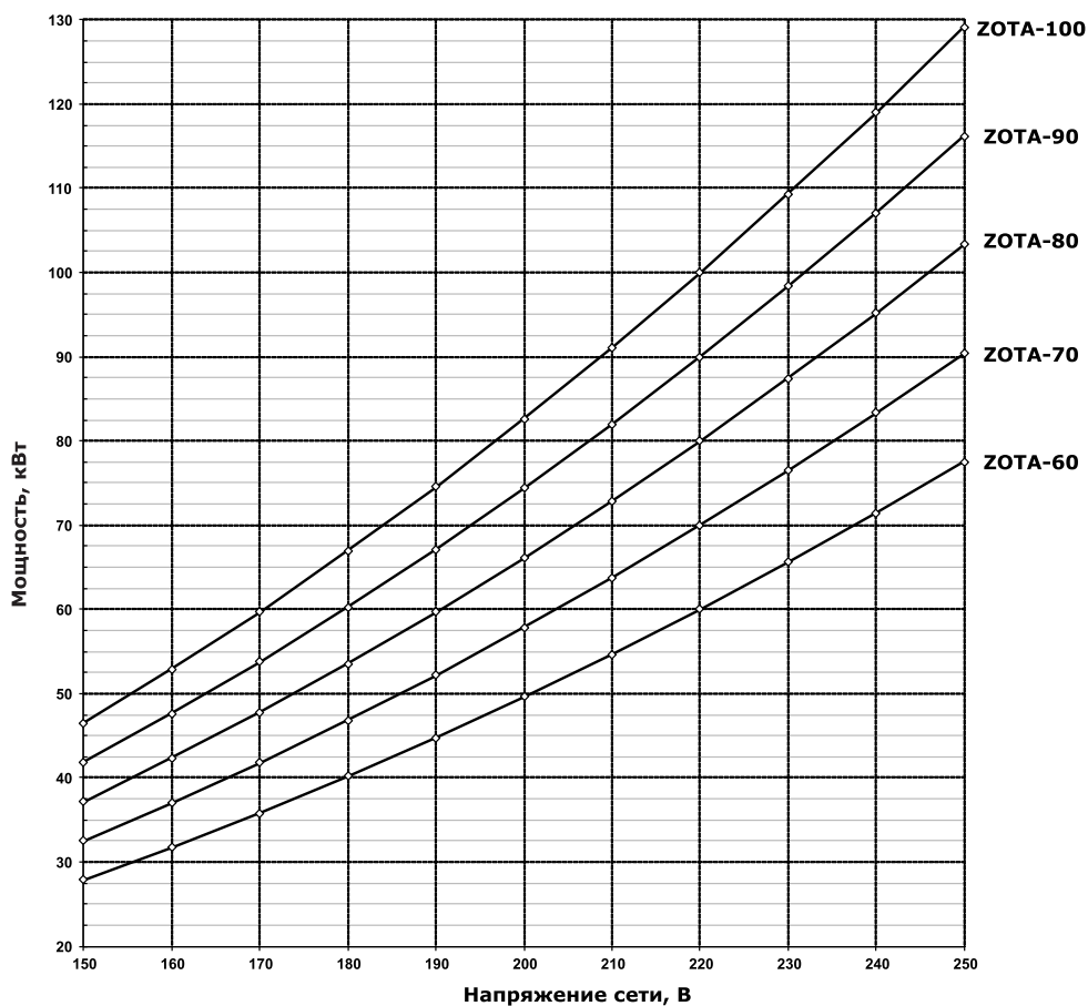
Рис.12 График изменения мощности электроводонагревателя в зависимости от питающего напряжения
