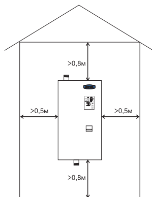
Рис.4 Схема установки электроводонагревателя
