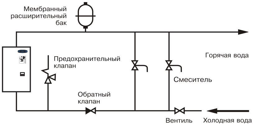
Рис.11 Упрощенная схема подключения в качестве электроводонагревателя с проточным режимом работы
