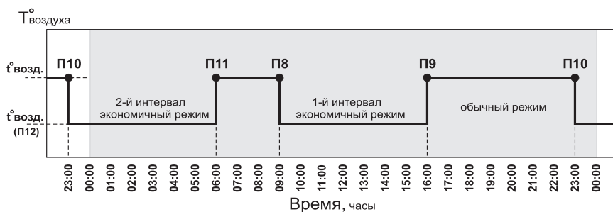
Рис.6 График температуры воздуха в помещении для Режим 1
