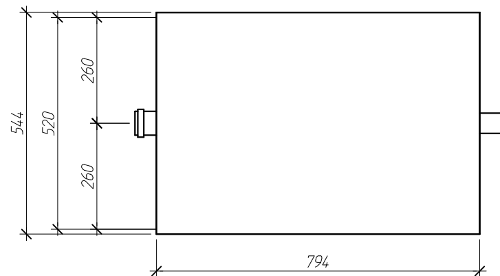
Вид сверху М 1:8
