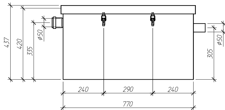
Вид спереди М 1:8
