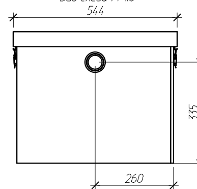
Вид слева М 1:8
