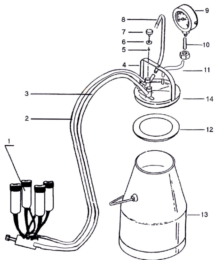
Монтажная схема №1
