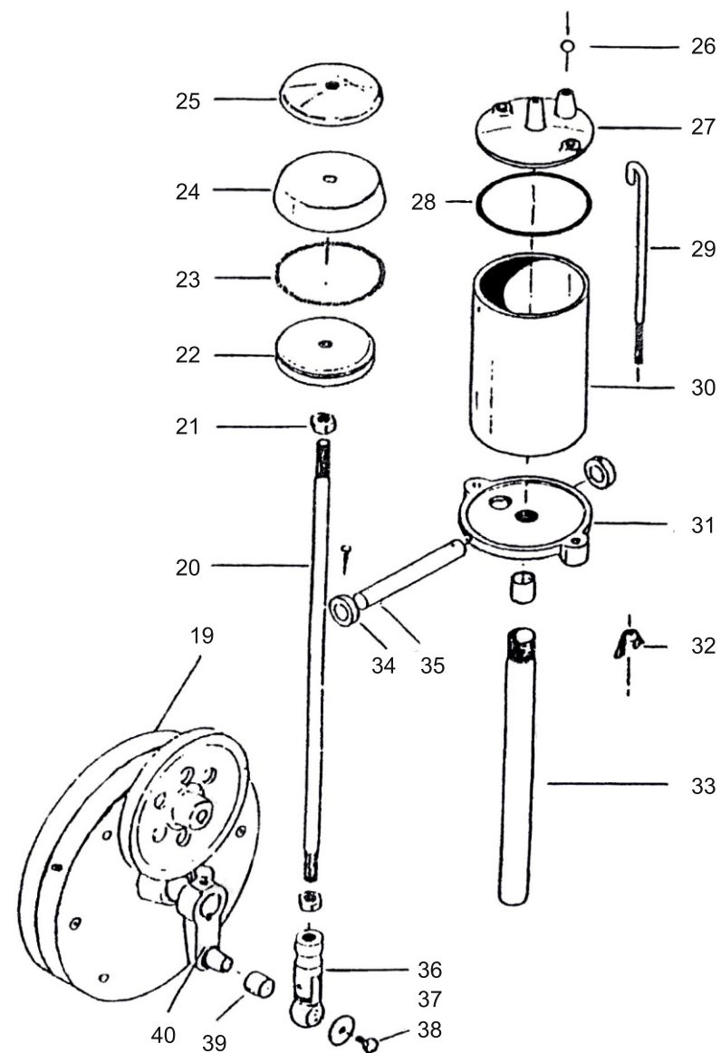
Монтажная схема №3
