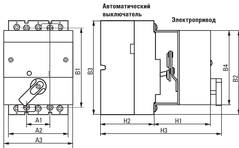
Рис. 3 Габаритные размеры приводов 125, 160
