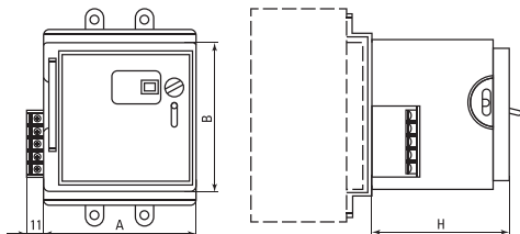
Рис. 4 Габаритные размеры приводов 250, 400, 800, 1600, CD/2
