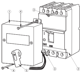
Рис. 5 Установка приводов 125А и 160А:
