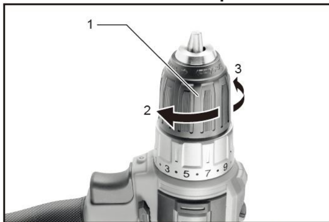
1. Муфта патрона 2. Зажать 3. Открыть
