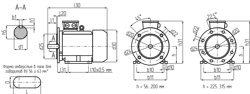
Рис. 2. Монтажное исполнение IM2081
