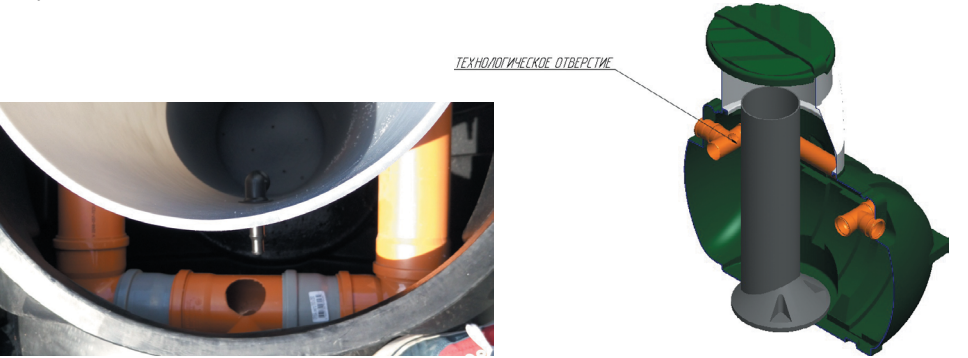
рисунок 2 Переливная система в стакане биофильтра «Rostok» Плюс
