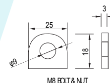
КЛЕММ T12
