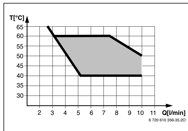
Рис 20 Диаграмма при температуре холодной воды на входе +15 °C
