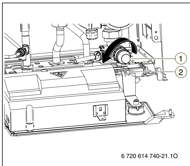
Рис 37 Предохранительный клапан
