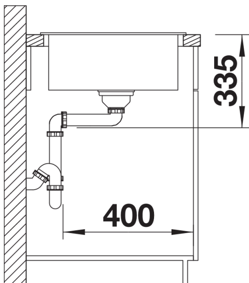
Вид сбоку
