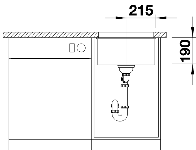
Вид спереди
