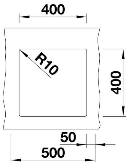
Вырез
