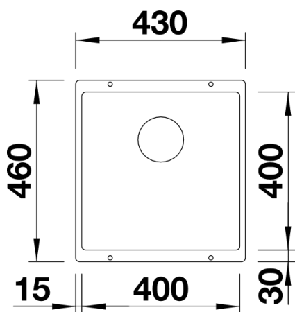
Вид сверху
