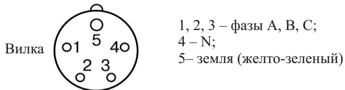
Рис. 2 Схема контактов на вилке
