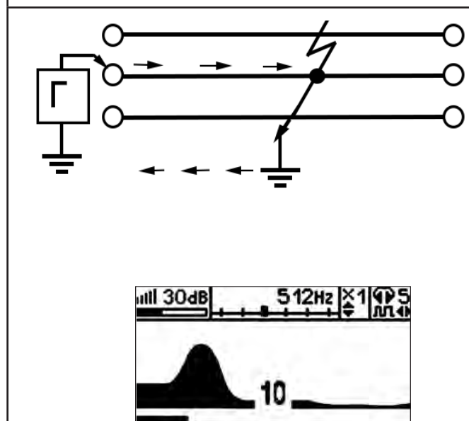
Рис.8.8 КЗ-однофазное
