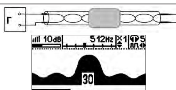
Рис.8.7 Муфта
