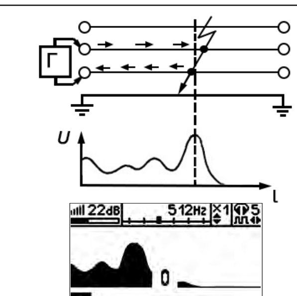
Рис.8.9 КЗ-двухфазное
