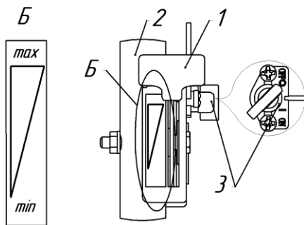
Рис.10 Дистанционное управление двигателем
