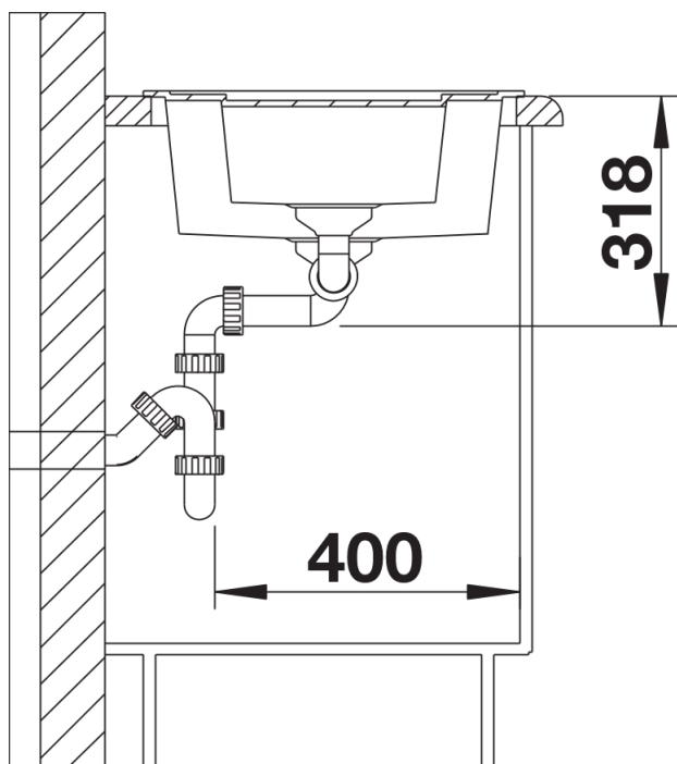
Вид сбоку
