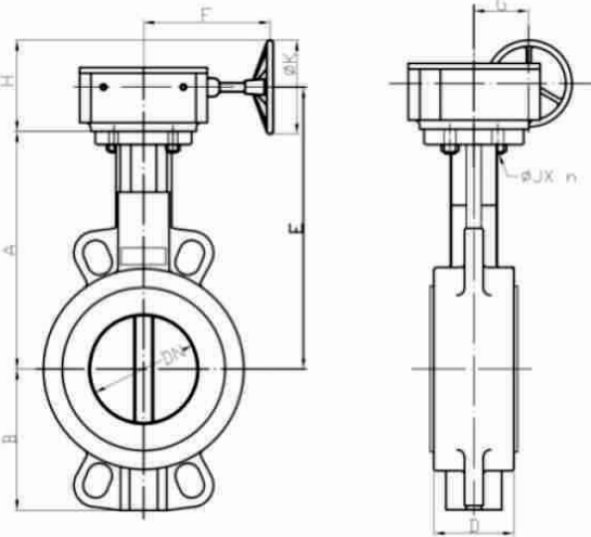
Редуктор DN 100 - 300
