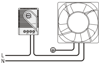
Рисунок 3. Схема подключения вентилятора с термостатом SQ0832-0021
