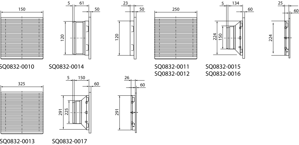
Рисунок 1. Габаритные размеры вентиляторов, мм
