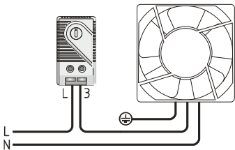
Рисунок 2. Схема подключения вентилятора с термостатом SQ0832-0019
