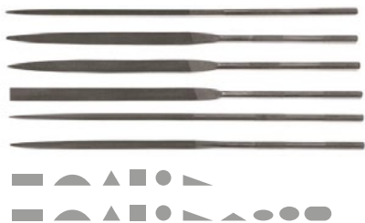
Набор надфилей LOM
