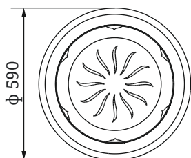
Рисунок 2. Габаритные размеры очага Неандерталь
