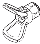
bez trysky závit F (11/16 – 16 UN) pro stříkací pistole Wagner Objednáací č. 0289391 bez trysky závit G (7/8 – 14 UN) pro stříkací pistole Graco/Titan Objednáací č. 0289390
