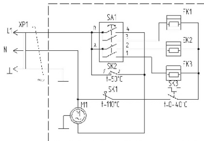
Схема электрическая QS 5; QSE 5020
