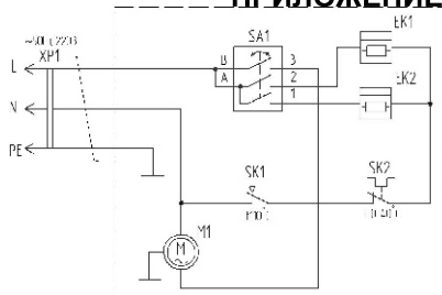
Схема электрическая QS 3; QSE 3020
