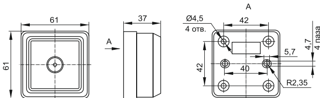
Рисунок 4 – Розетки телевизионные: РТВ20-ОБ, РТВ20-ОКм, РТВ20-ОС, РТВ20-ОД
